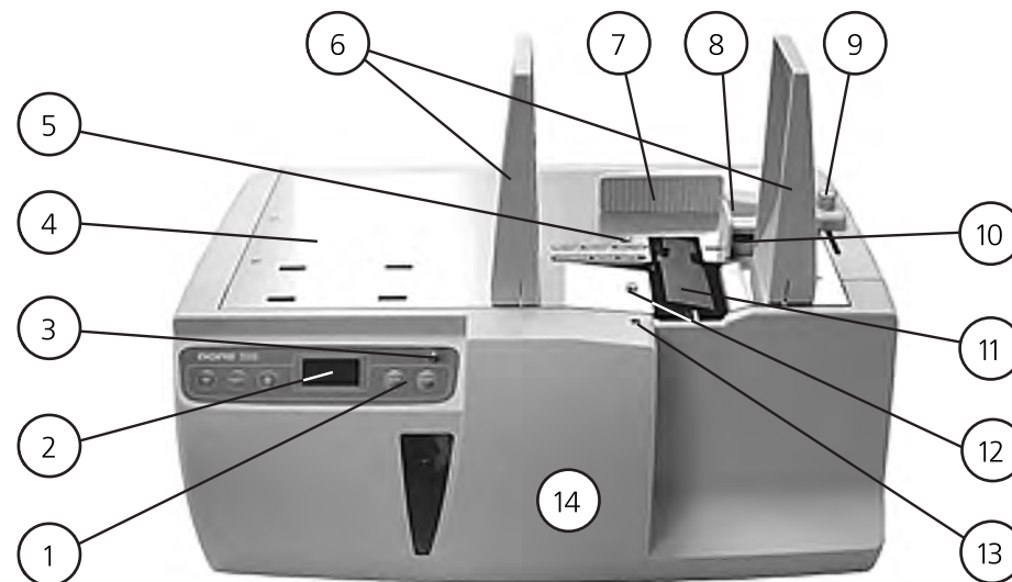
Рисунок 1 Вид спереди
